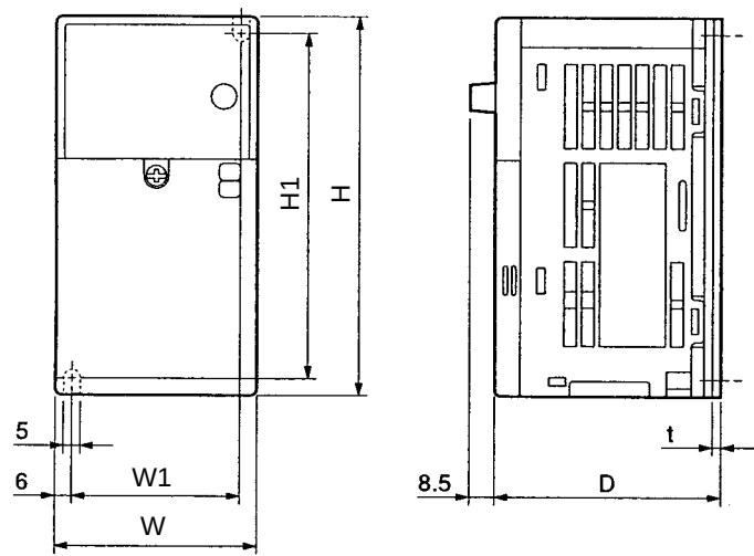
Modello con alimentazione mono/trifase a 220 Vc.a.
