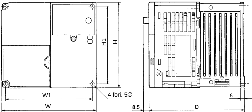
Modello con alimentazione mono/trifase 220 Vc.a.
